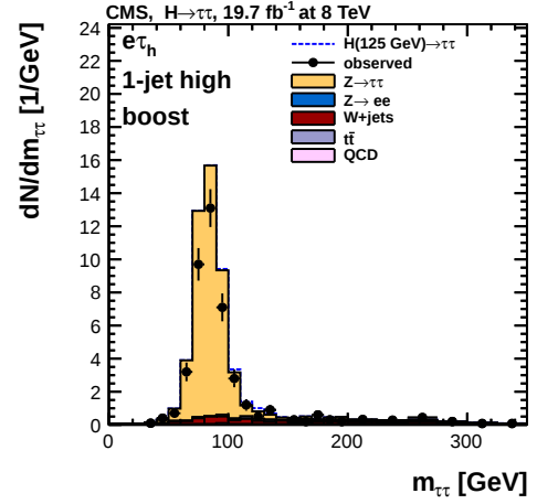
(d) SVfit Mass : e\tau_h 1-jet high \uparrow
