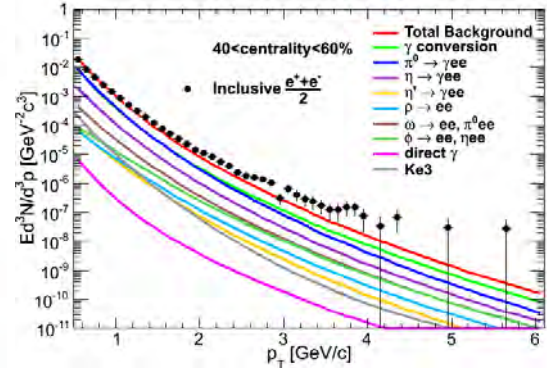
(d) Centrality 40-60%
