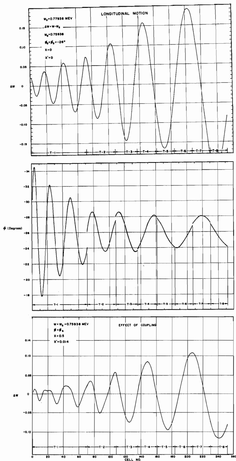
Fig. 21 LONGITUDINAL MOTION
