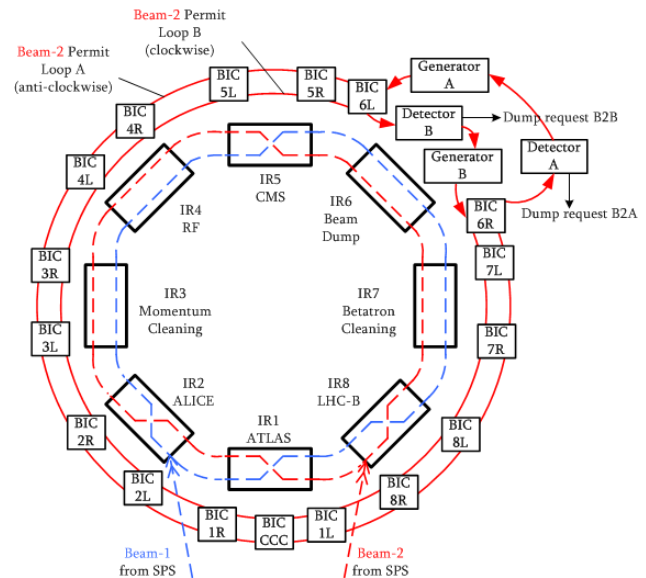
Figure 1: BIS layout for Beam 2.
