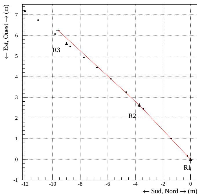
FIG. 5.9: Vue de haut de la ligne. Les triangles représentent les distance-mètres et les points indiquent la position des inclinomètres. Les segments illustrent le positionnement de la ligne, établi d'après les données acoustiques. On observe un décalage entre les données des inclinomètres et les résultats de la méthode acoustique (inférieur à 0.5 m); ceci est probablement dû au fait que les prises de données n'ont pas été simultanées.
