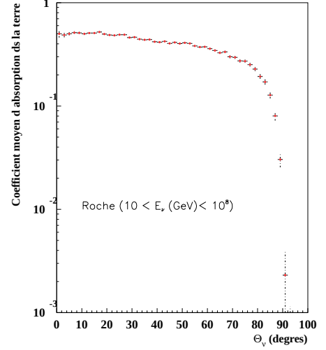
FIG. 2.8: Effet moyen de l'absorption de neutrinos d'énergie 10 < E_{\nu} (GeV) < 10 8 en fonction de leur angle zénithal d'incidence.
