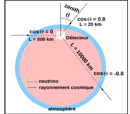
FIG. 1.14: Représentation schématique de la détection de neutrinos atmosphériques.
