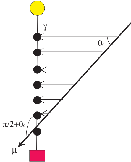
FIG. 7.9: Une trace de muon avec un angle zénithal de \frac{\pi}{2} + \theta_c illumine les photomultiplicateurs simultanément.
