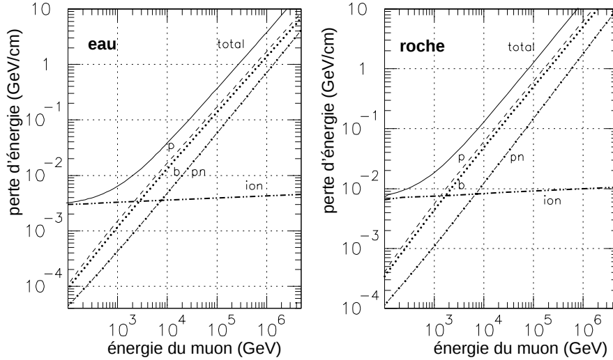
FIG. 2.11: Contribution à la perte d'énergie des principaux types de processus radiatifs engendrés par le passage d'un muon dans l'eau (gauche) et dans la roche (droite)
