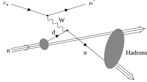
FIG. 2.1: Diagramme de Feynman de l'interaction d'un neutrino muonique sur neutron par courant chargé.
