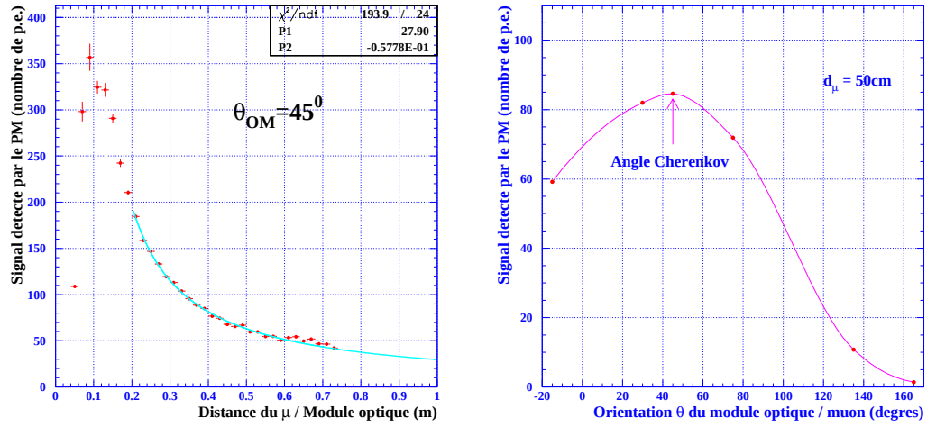
FIG. 2.32: L'histogramme de gauche représente le nombre de photo-électrons détectés en fonction de la distance à la trace lorsque l'angle entre celle-ci et le module optique est de 45 degrés. Compte tenu des dimensions de la gamelle, les données ne sont disponibles que pour un éloignement maximal de 70 cm. Le schéma montre une extrapolation jusqu'à un mètre. L'histogramme de droite représente le nombre de photo-électrons détectés en fonction de l'angle formé par la direction de visée du module optique et la direction du \mu incident, pour des traces éloignées de 50 cm de la photo-cathode. Un maximum est atteint vers 43 degrés (angle Tcherenkov dans l'eau), c'est à dire lorsque la direction du photon est parallèle à l'axe du photo-tube.
