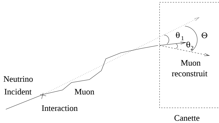
FIG. 3.3: Représentation schématique de la méthode de génération des événements simulés. Après l'interaction du neutrino, le muon induit est propagé jusqu'à la canette en tenant compte des diffusions multiples le long de son parcours.
