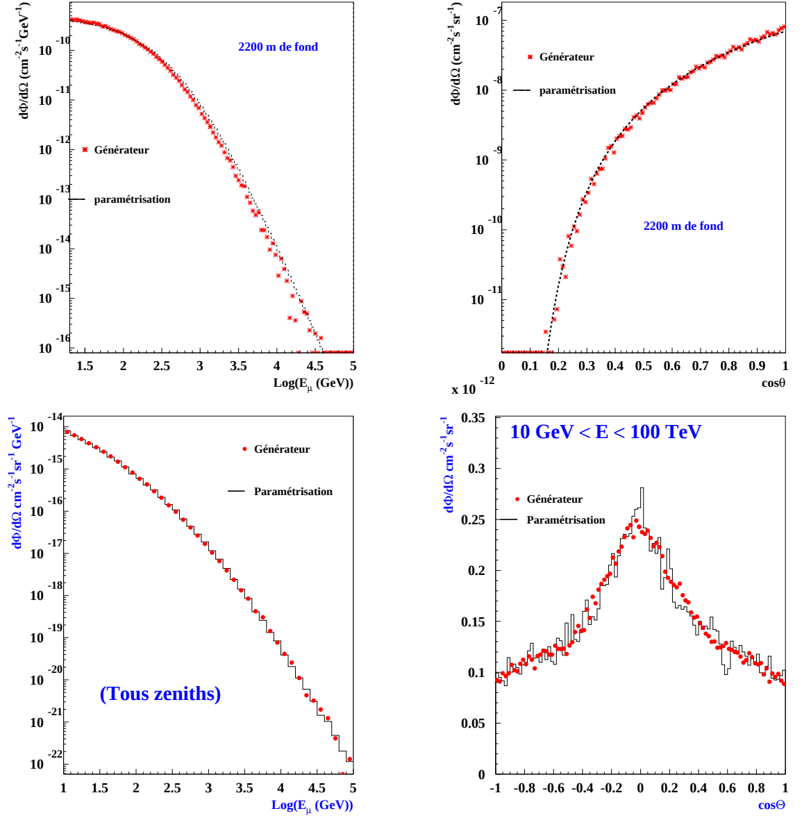
FIG. A.2: Comparaison entre les résultats du générateur sur tout le domaine utile en énergie et en direction, et les paramétrisations initiales sur la base desquelles il a été développé. Les deux figures du haut ont trait aux muons atmosphériques, à 2200 m de fond, celles du bas correspondent aux muons issus de neutrinos atmosphériques.
