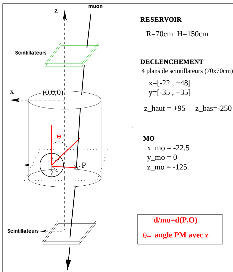
FIG. 2.31: Dispositif de test : la «gamelle»
