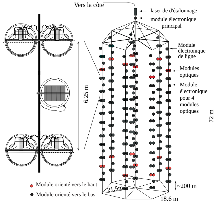
FIG. 2.19: Schéma du détecteur Baïkal. Certains modules optiques sont orientés vers le haut, ce qui permet ainsi l'établissement d'un meilleur veto pour rejeter le bruit de fond. Le détecteur est largement exposé aux salissures en suspension dans le lac, mais la couche de glace qui se forme chaque hiver permet de récupérer les lignes et de nettoyer les modules optiques.
