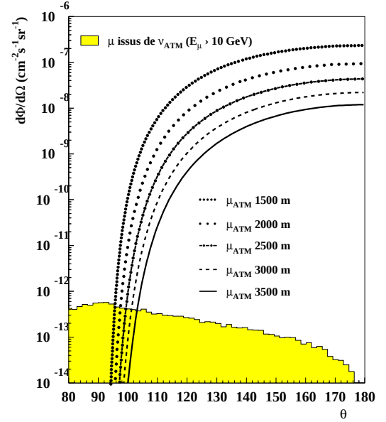
FIG. 2.18: Evolution du bruit de fond suivant la profondeur
