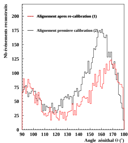
FIG. B.12: Distribution brute des angles zénithaux des événements reconstruits pour l'alignement n°1 et l'alignement n°2. Ici l'angle zénithal est restreint à l'intervalle [90, 180] . Les deux alignements permettent de recentrer les résidus mais les résultats à la reconstruction sont très différents. L'alignement n°2, plus fiable, fournit le meilleur accord avec les simulations.
