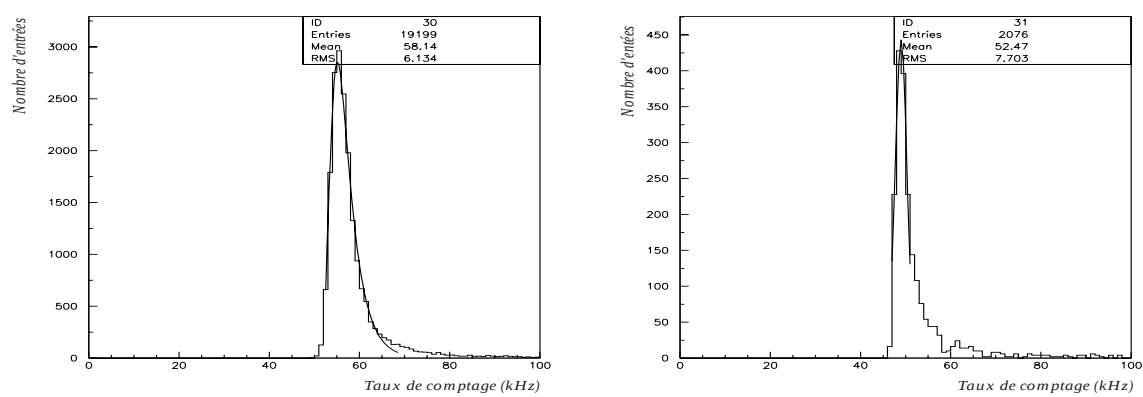
FIG. 5.16: Taux de comptage moyen lors d'une journée (à droite) et d'une nuit (à gauche) pour un PM de 10"
