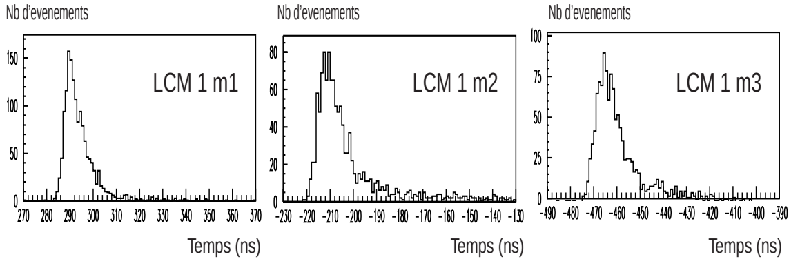
FIG. 6.14: Réponse temporelle des photomultiplicateurs du LCM 1 sous illumination de la LED du module optique de plus grande altitude de la ligne. L'asymétrie observée dans les distributions est essentiellement due à la diffusion.
