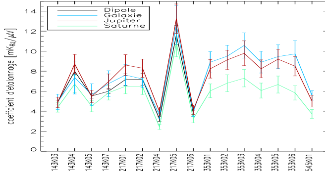
FIG. 11.6: Coefficient d'étalonnage pour les bolomètres d'Archeops. Toutes les sources d'étalonnage sont superposées : le dipôle cosmologique (en noir), la Galaxie (en bleu), Jupiter (en rouge) et Saturne (en vert). Les barres d'erreurs tiennent compte des erreurs de mesure et des erreurs absolues.
