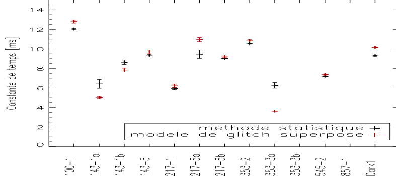
FIG. 8.5: Comparaison des constantes de temps des bolomètres du CQM estimées à l'aide de la méthode statistique en noir et du modèle de glitchs superposés en rouge. Mis à part le 353-3a, les méthodes sont en bon accord.
