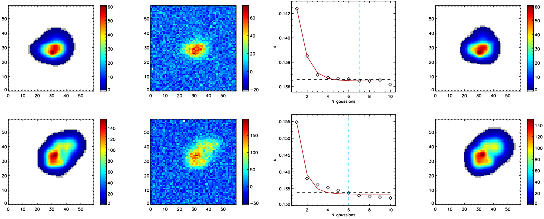
FIG. 10.2: Décomposition du lobe avec ASYMPFAST pour la simulation 1 (en haut) et la simulation 2 (en bas) avec 10% de bruit. De gauche à droite : la simulation de lobe ; la simulation de lobe avec 10% de bruit ; la dispersion quadratique S en fonction de N (la ligne rouge représente l'ajustement exponentiel et la ligne bleue le nombre de gaussiennes retenu pour la décomposition) ; la reconstruction à partir de N = 7 et 8 gaussiennes.
