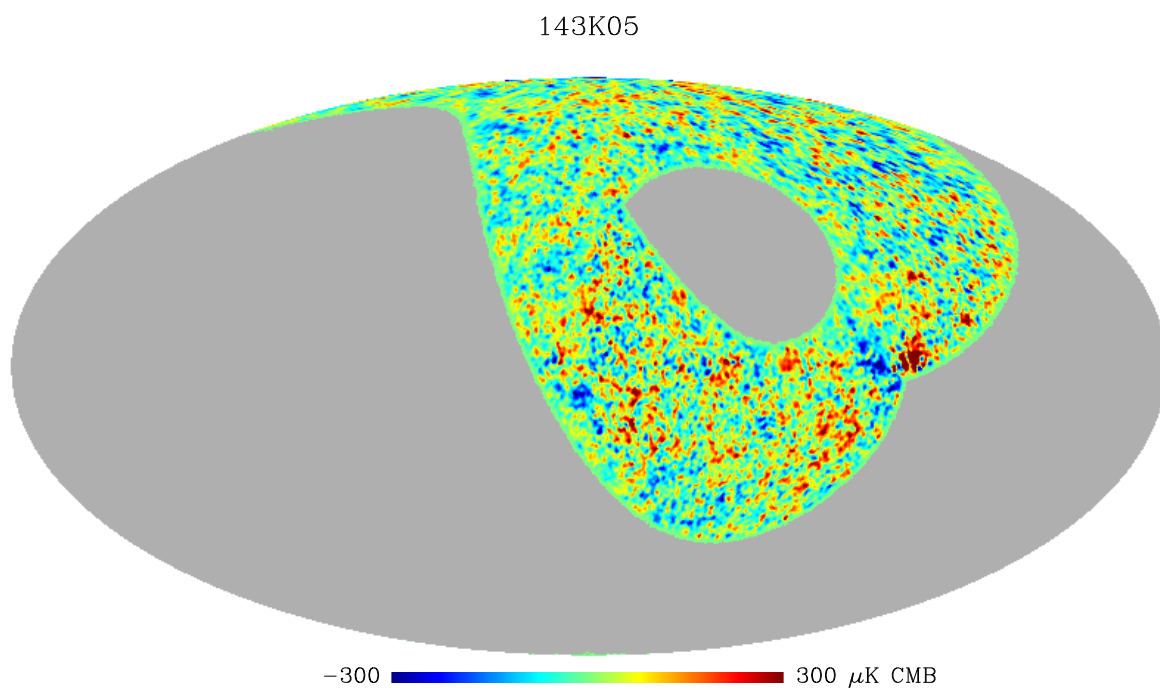
FIG. B.3: Carte des anisotropies vues par le détecteur 143K05 à la résolution de N_{side} = 256 et lissée par une gaussienne de 1 degré.
