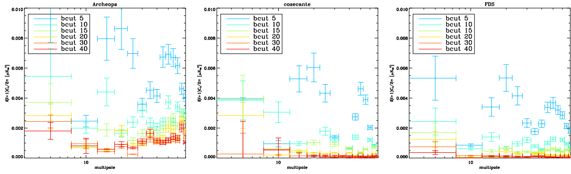
FIG. 18.3: Spectres de puissance en température pour Archeops, un modèle en cosécante et les données FDS. De gauche à droite : spectre d'Archeops à 353 GHz ; spectre du modèle en loi de cosécante I(b) \propto 1/\sin(b) normalisée sur l'amplitude des cartes FDS ; spectre des données FDS. Les spectres sont présentés pour différentes coupures galactiques ( |b| > 5, 10, 15, 20 et 30 ).
