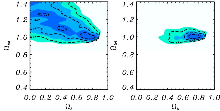
FIG. 22.2: Estimation des paramètres \Omega_{tot} et \Omega_\Lambda avec Archeops et les autres expériences CMB (à gauche). À droite : avec la valeur de H_0 donnée par le HST.
