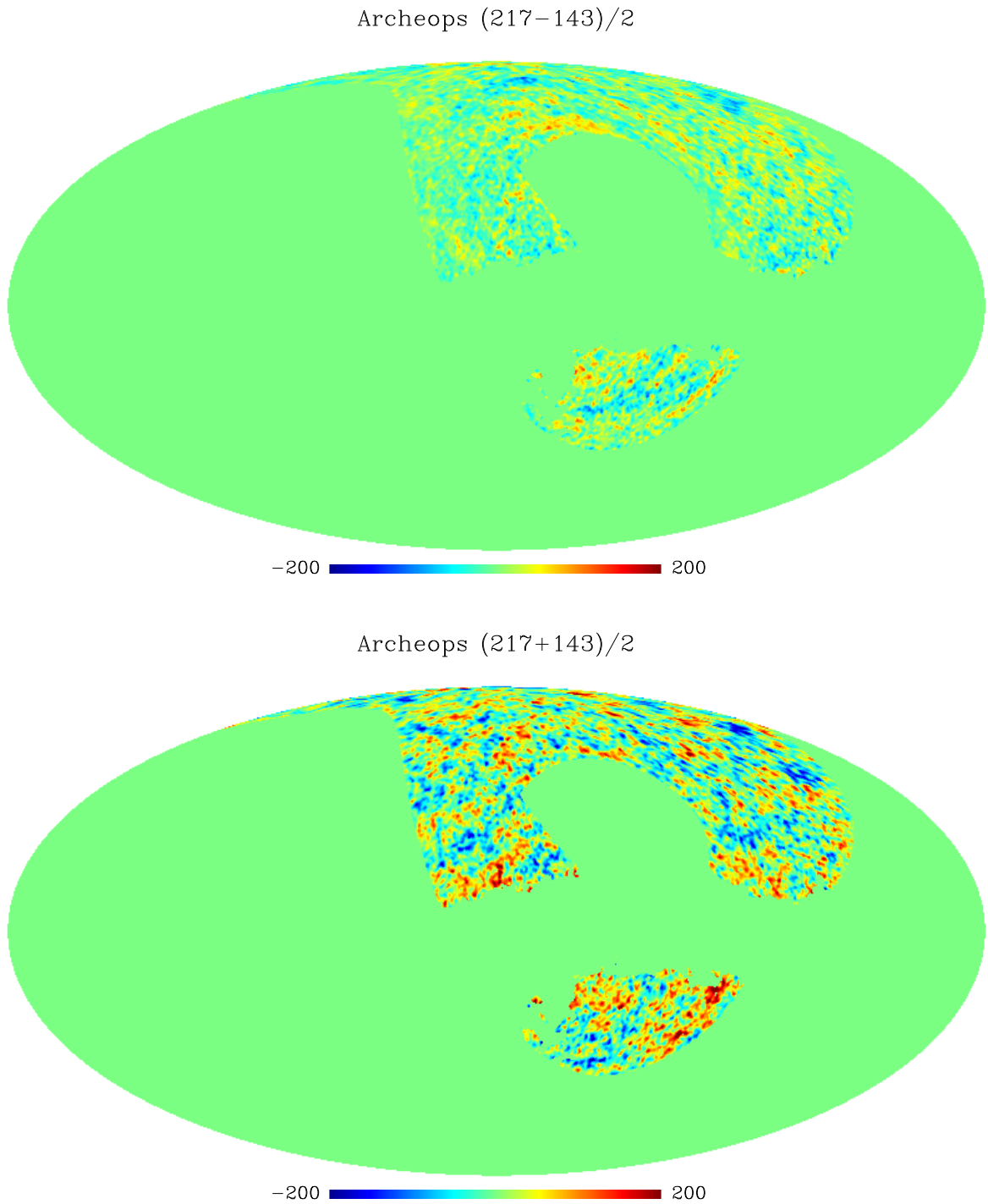
FIG. 19.1: Cartes demi-différence et demi-somme du CMB d'Archeops à 143 et 217 GHz. Les cartes sont la combinaison des 4 (resp. 2) bolomètres les plus sensibles à 143 et 217 GHz. En haut : demi-différence 143-217, en bas : demi-somme 143+217. Le rapport signal sur bruit est de 1.9. La demi-différence présente des résidus atmosphériques (à haute latitude) et galactiques (essentiellement dans l'hémisphère Sud).
