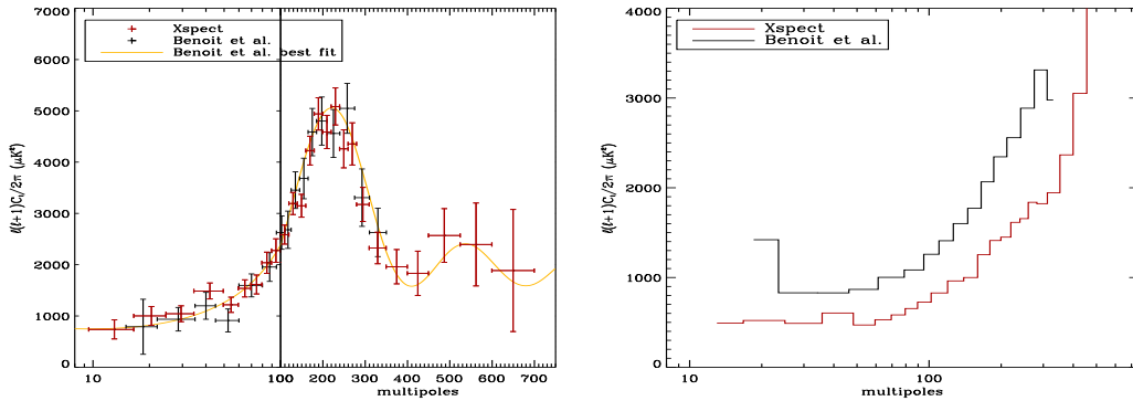
FIG. 16.16: Comparaison entre les deux estimations du spectre de puissance angulaire du CMB d'Archeops . à gauche : comparaison des spectres. À droite : comparaison des barres d'erreur.
