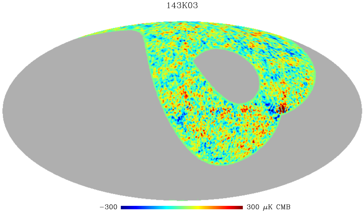
FIG. B.1: Carte des anisotropies vues par le détecteur 143K03 à la résolution de N_{side} = 256 et lissée par une gaussienne de 1 degré.
