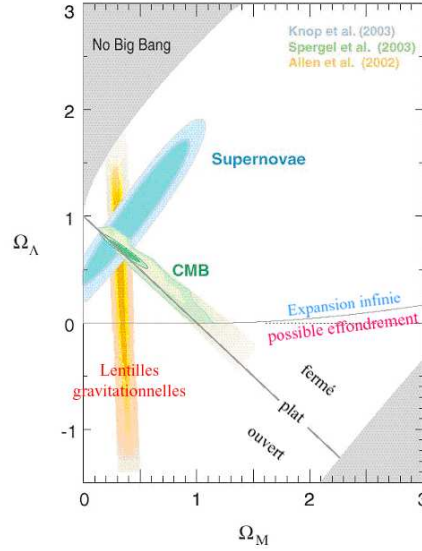
FIG. 2.9: Contraintes dans le plan ( \Omega_M, \Omega_\Lambda ) apportées par le CMB, les supernovae de type Ia et les lentilles gravitationnelles. CMB et supernovae permettent de contraindre \Omega_\Lambda \simeq 0.7 et \Omega_M \simeq 0.3 .
