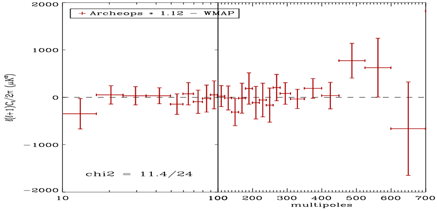
FIG. 19.7: Différence entre le spectre croisé Archeops/WMAP et celui de WMAP sur la couverture Archeops. Le spectre croisé est multiplié par un facteur 1.12 en température. Le \chi^2 est de 11.4/24. Les erreurs tiennent compte de la variance d'échantillonnage.
