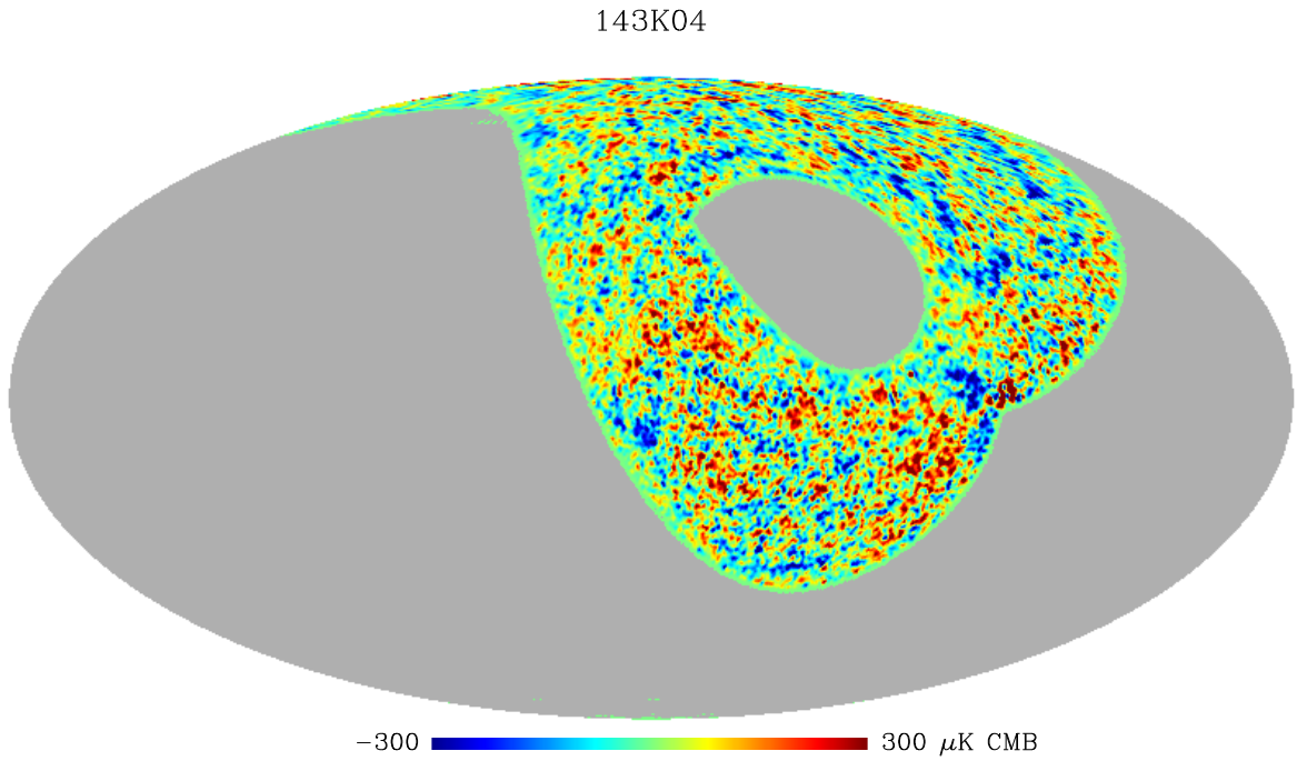
FIG. B.2: Carte des anisotropies vues par le détecteur 143K04 à la résolution de N_{side} = 256 et lissée par une gaussienne de 1 degré.
