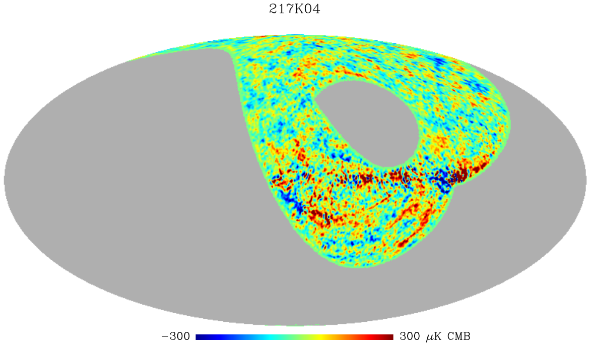
FIG. B.5: Carte des anisotropies vues par le détecteur 217K04 à la résolution de N_{side} = 256 et lissée par une gaussienne de 1 degré.
