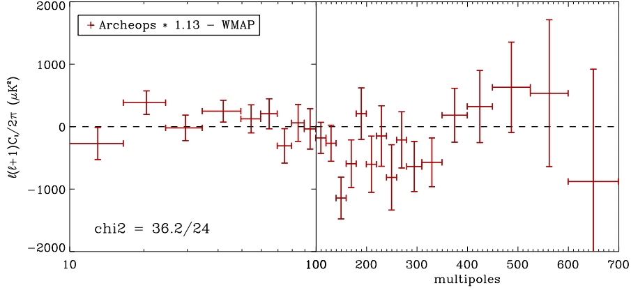
FIG. 19.5: Différence entre les spectres de WMAP et Archeops sur la couverture Archeops. Le spectre d'Archeops est multiplié par un facteur 1.06 \pm 0.01 en température. Le \chi^2 est de 36.2/24. Les erreurs tiennent compte de la variance d'échantillonnage.
