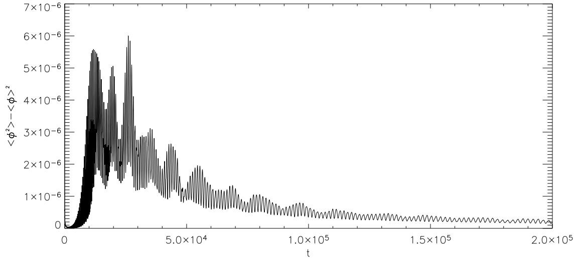
FIG. 4.3: Variance du champ scalaire pendant la phase de reheating. La variance augmente exponentiellement pendant la phase de résonance jusqu'à Var(\phi) \simeq 5 \cdot 10^{-6} m_P^2 .
