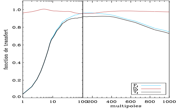
FIG. 16.3: Fonctions de transfert des filtres estimées par simulations. en bleu : la fonction de filtrage F_\ell , en rouge : la fonction de déstriage D_\ell , en noir : la fonction totale T_\ell . Comme le filtrage est le même, on utilise la même fonction pour tous les bolomètres.
