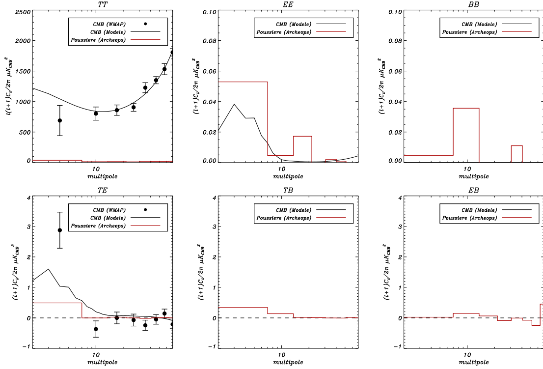
FIG. 20.2: Spectres de puissance angulaire de la poussière extrapolés aux fréquences de WMAP et comparés aux spectres de puissance du CMB (en noir). Les spectres de poussière d'Archeops à 353 GHz ont été extrapolés avec une loi de puissance d'indice spectral 1.7. A grande échelle angulaire ( 2 \leq \ell \leq 7 ), l'amplitude du spectre de poussière TE atteint 0.49 \pm 0.10 comparée aux C_\ell^{TE} = 2.87 \pm 0.59 \mu\text{K}_{\text{CMB}}^2 . Le même point pour le spectre TB vaut 0.34 \pm 0.11 .
