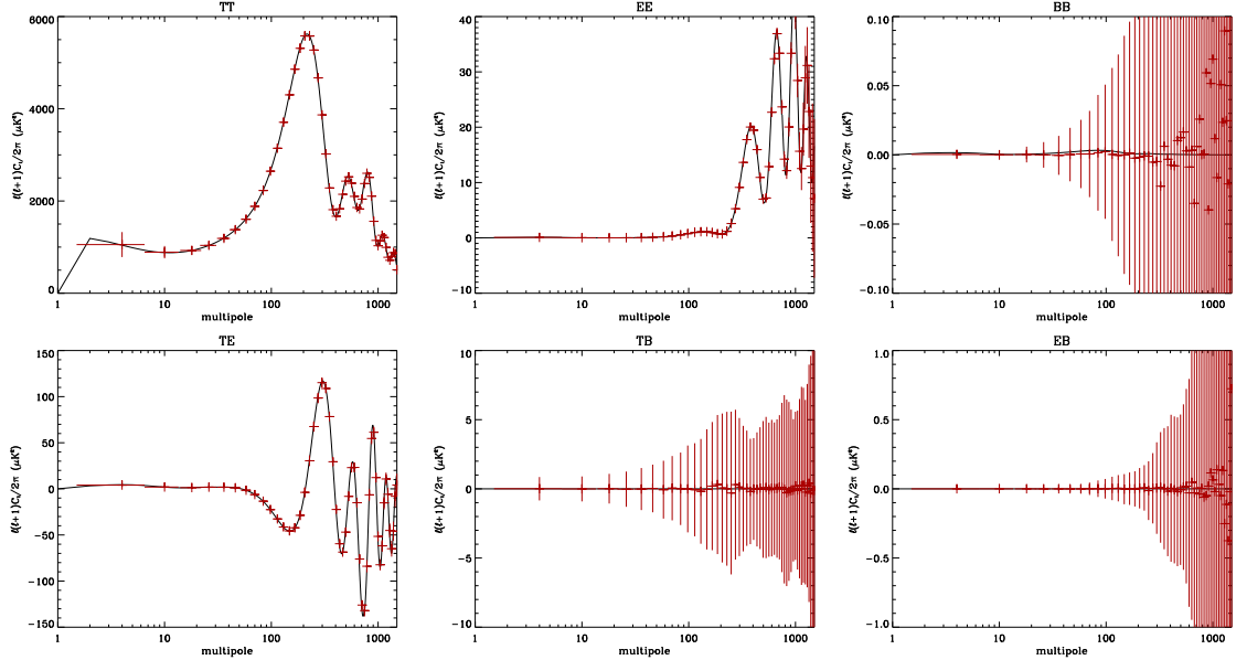
FIG. 17.2: Spectres de puissance angulaire du CMB pour Planck calculés avec XPOL. En haut : les spectres en température C_\ell^{TT} et en polarisation C_\ell^{EE} et C_\ell^{BB} . En bas : les spectres C_\ell^{TE} , C_\ell^{TB} et C_\ell^{EB} . Le modèle (en noir) est issu de celui de WMAP [Spergel et al. 2003] avec r = 0.05 .
