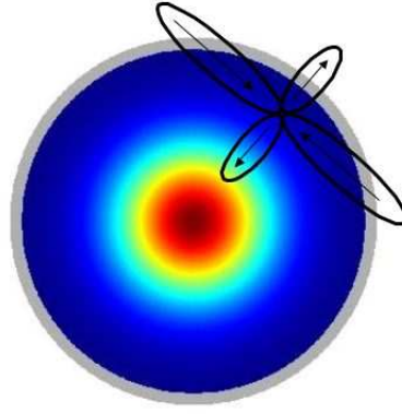
FIG. 2.4: Formation des anisotropies quadripolaires autour d'une sur-densité de matière. Les électrons le long du rayon de la sur-densité s'éloignent, alors que ceux qui appartiennent au même isocontour de densité se rapprochent.
