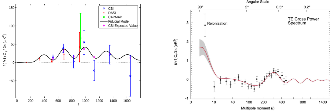
FIG. 2.11: A gauche : mesures du spectre polarisé E par les expériences DASI [Leitch et al. 2004], CBI [Readhead et al. 2004] et CAPMAP [Barkats et al. 2005]. La figure est issue de [Readhead et al. 2004]. A droite : spectre corrélé T-E de WMAP [Kogut et al. 2003]
