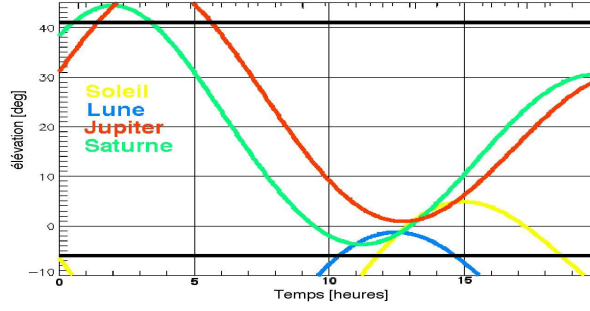
FIG. 11.1: Ephéméride des principales sources pendant le vol KS3 Archeops. L'élévation de la source est tracée en fonction du temps à partir du début du vol. Pendant la nuit polaire la Lune et le Soleil restent sous l'horizon. Archeops, situé à 35 km d'altitude et pointant à élévation constante (41 degrés trait noir ), est sensible aux sources lorsqu'elles dépassent -6 degrés d'élévation ( trait noir ). Les planètes Saturne en vert et Jupiter en rouge sont vues deux fois en début de vol.
