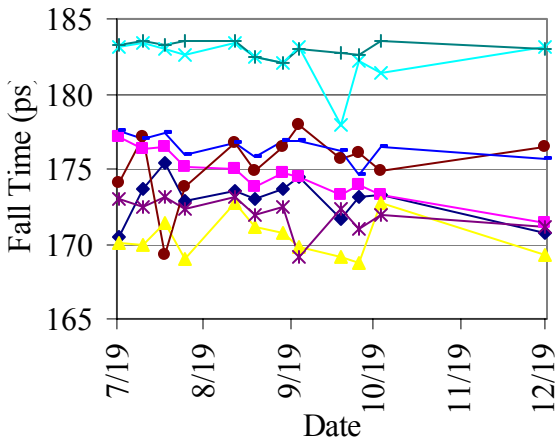
Fig. 3.3 Fall Time
