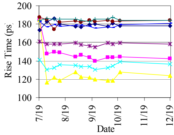
Fig. 3.4 Rise Time
