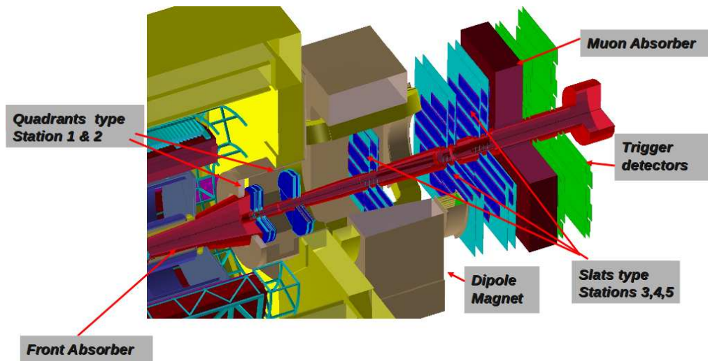
Figure 2.20 – Vue du spectromètre à muons.
