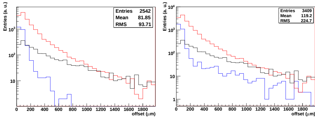
Figure 6.9 – Offset des muons provenant de la désintégration d’un méson B (noire), d’un méson D (rouge), d’un \phi en bleu (figure de gauche) et d’un J/\psi en bleu (figure de droite) pour des pixels de 20 \mu\text{m} par 20 \mu\text{m} et 150 \mu\text{m} d’épaisseur.
