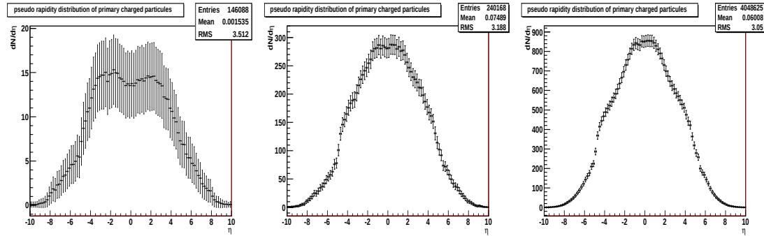
Figure 6.17 – Multiplicité en fonction de la pseudo-rapacité dans la simulation pp (gauche), Pb-Pb périphérique (centre), et Ca-Ca (droite).
