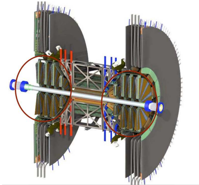
Figure 5.7 – Illustration du nouveau détecteur à vertex (VTX + FVTX) dans l'expérience PHENIX [137].
