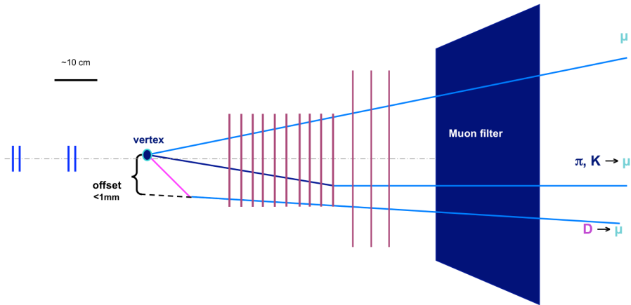
Figure 5.4 – . Vue schématique du télescope de NA60. Illustration du concept d'offset [135].
