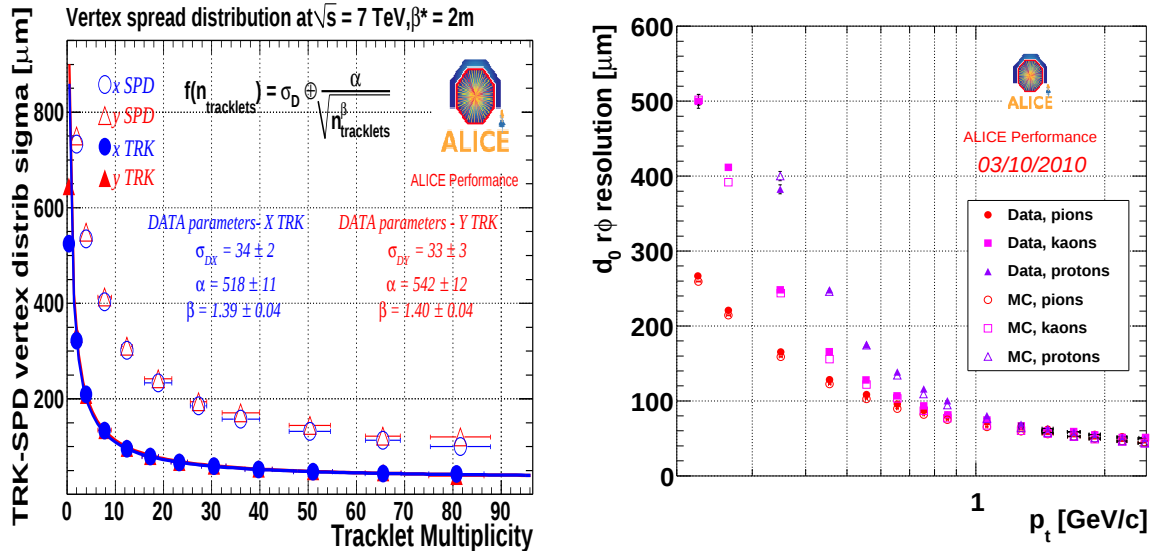
Figure 2.14 – Gauche : distribution de la dispersion du vertex primaire reconstruit avec les traces de l'ITS complet (TRK) ou avec le SPD seul (SPD) en collisions pp à \sqrt{s} = 7 \text{ TeV} . La limite asymptotique estime la taille de la région lumineuse, vue par les vertex reconstruits avec les traces. Droite : estimation de la résolution sur le paramètre d'impact transverse, obtenue à partir de traces qui satisfont aux coupures standards de la TPC, et présentent 2 points dans le SPD [73].
