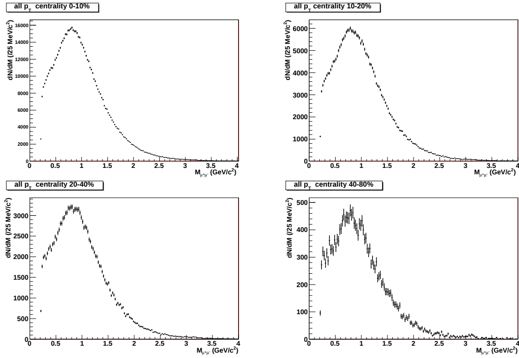
Figure 4.12 – Spectre en masse invariante des dimuons de signes opposés pour la tranche en centralité 0-10% (en haut à gauche), pour la tranche en centralité 10-20% (en haut à droite), pour la tranche en centralité 20-40% (en bas à gauche) et pour la tranche en centralité 40-80% (en bas à droite).
