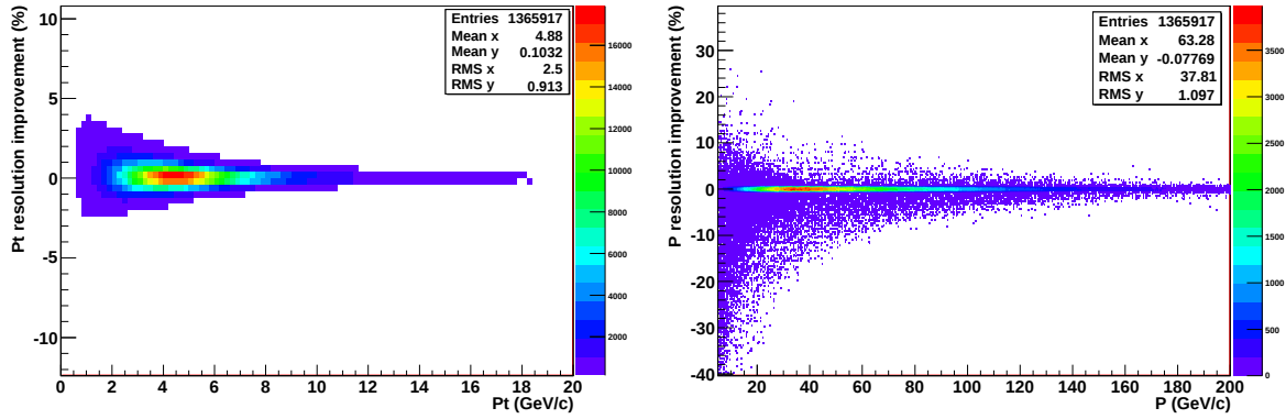
Figure 6.10 – Amélioration de la résolution sur la détermination de l'impulsion transverse (gauche) et de l'impulsion totale (droite) pour chaque muon détecté dans le spectromètre.
