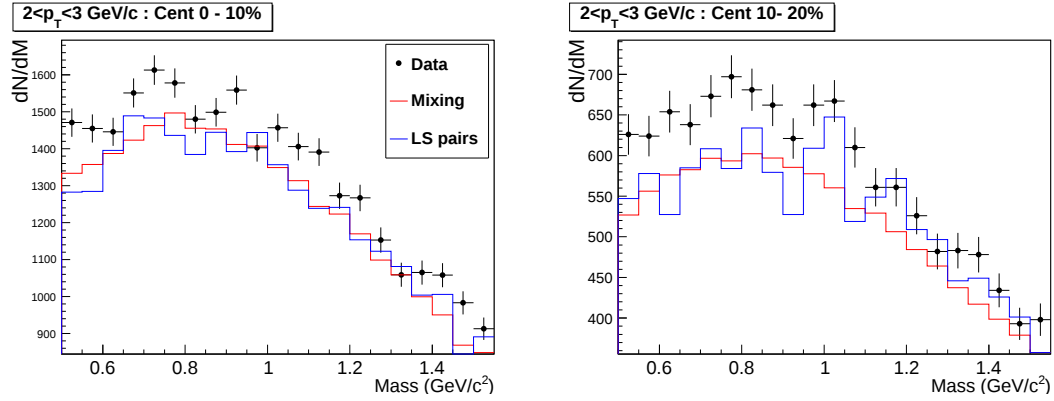
Figure 4.21 – Spectre en masse invariante des dimuons de signes opposés pour une impulsion transverse du muon simple supérieure à 0.5 GeV/c et une impulsion du dimuon comprise entre 2 et 3 GeV/c, pour les centralités 0-10% (à gauche) et 10-20% (à droite). Les 2 coupures en impulsion sont appliquées au niveau des chambres de trajectographie.
