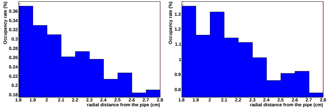
Figure 5.25 – Taux d’occupation dans le premier plan de pixels au plus proche de l’IP, et dans les premiers millimètres au plus proche du faisceau (à gauche pour des pixels de 50\ \mu\text{m} par 50\ \mu\text{m} et à droite pour des pixels de 100\ \mu\text{m} par 100\ \mu\text{m} ), avec une simulation tuyau conique.
