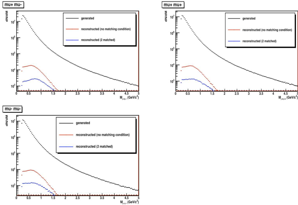
Figure 3.20 – Spectres en masse invariante générés (courbe noire) et reconstruits dans le cas où aucun muon n'est associé avec une trace dans les chambres de déclenchement (courbe rouge), ou dans le cas où les deux muons ont laissé une trace dans les chambres de déclenchement (courbe bleue) pour les dimuons de signes opposés (en haut à gauche) et pour les dimuons de même signe ( \mu^+\mu^+ en haut à droite et \mu^-\mu^- en bas à gauche).
