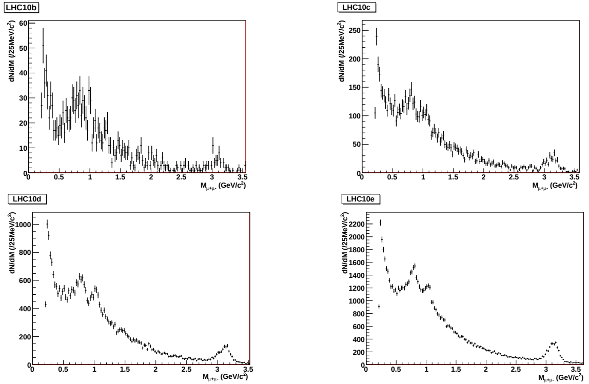
Figure 3.11 – Spectres en masse invariante des dimuons pour la période b (en haut à gauche), pour la période c (en haut à droite), pour la période d (en bas à gauche) et pour la période e (en bas à droite).
