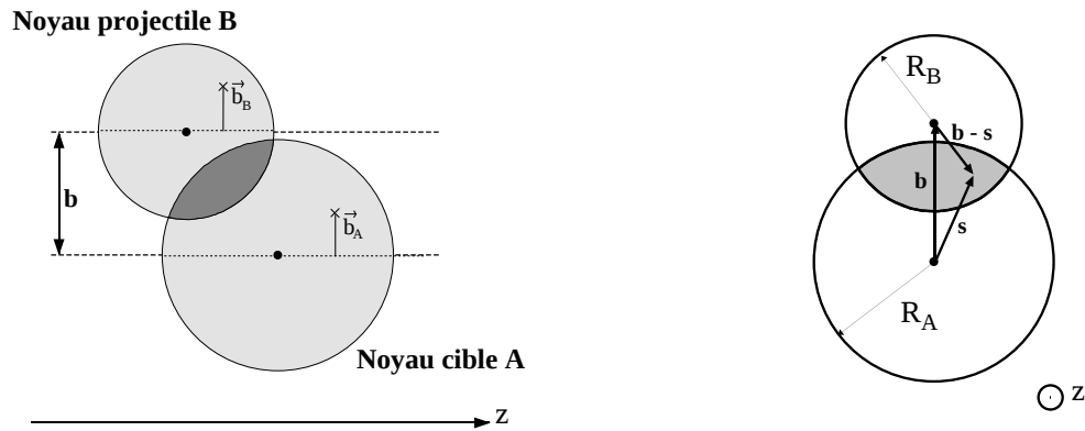
Figure 6.36 – Représentation schématique d'une collision entre deux noyaux A et B avec un paramètre d'impact \vec{b} suivant l'axe longitudinal (gauche) et dans le plan transverse (droite).
