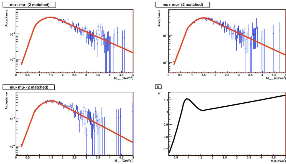
Figure 3.21 – Courbes d’acceptance ( \times efficacité) pour les dimuons de signes opposés (en haut à gauche), pour les dimuons \mu^+\mu^+ (en haut à droite), pour les dimuons \mu^-\mu^- (en bas à gauche) dans le cas où les deux muons ont laissé une trace dans les chambres de déclenchement. La courbe en bas à droite correspond au calcul du facteur R .
