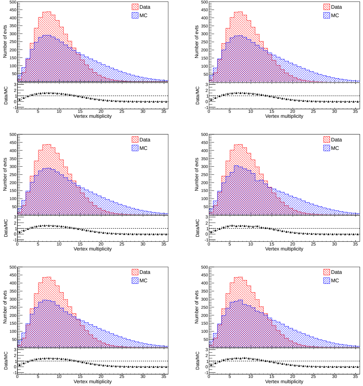
FIG. 7.9 – Distribution du nombre de vertex générés pour les fonds MC et facteurs de corrections, de haut en bas en partant de la gauche, t\bar{t} issus du MS, W +jets, Z +jets, top canal-s, top canal-t et top canal-tW.
