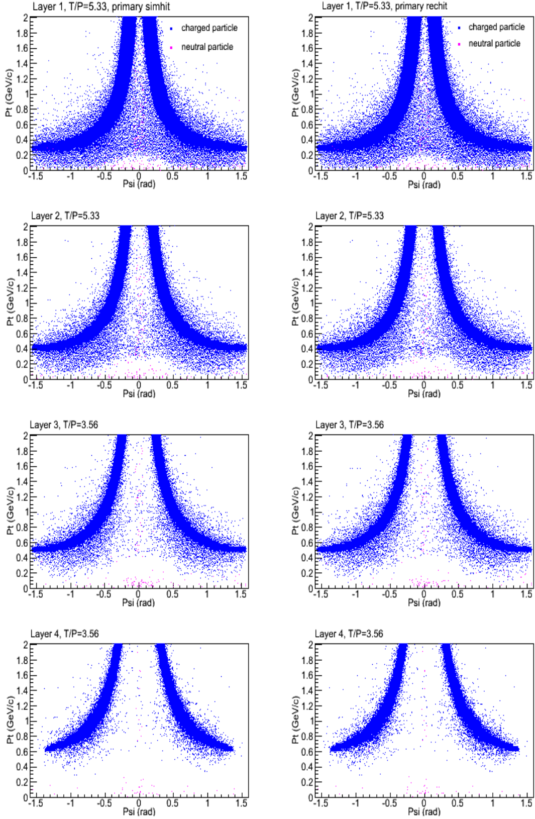
FIG. 6.19 – Distribution, agrandie entre 0 et 2 \text{ GeV} \cdot c^{-1} , des amas primaires issus d'événements de biais minimum simulés (colonne de gauche) et reconstruits (colonne de droite), en fonction de \psi pour chaque couche.
