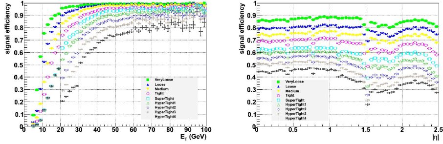
FIG. 7.11 – Efficacités de l’algorithme d’identifications des électrons (CiC), pour différentes valeurs de coupures, en fonction de l’énergie transverse (figure de gauche) et de l’angle \eta (figure de droite).
