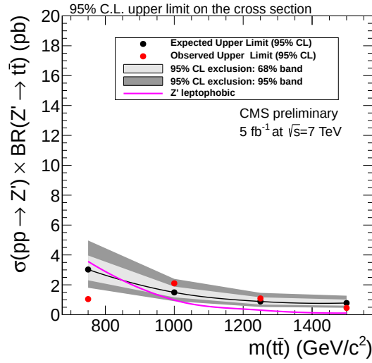
FIG. 8.7 – Courbe de limite de la section efficace de production de nouvelle physique pour les quatre hypothèses de masse (750, 1000, 1250 et 1500 \text{GeV}.c^{-2} ). La courbe théorique est issue de l'article [135]
