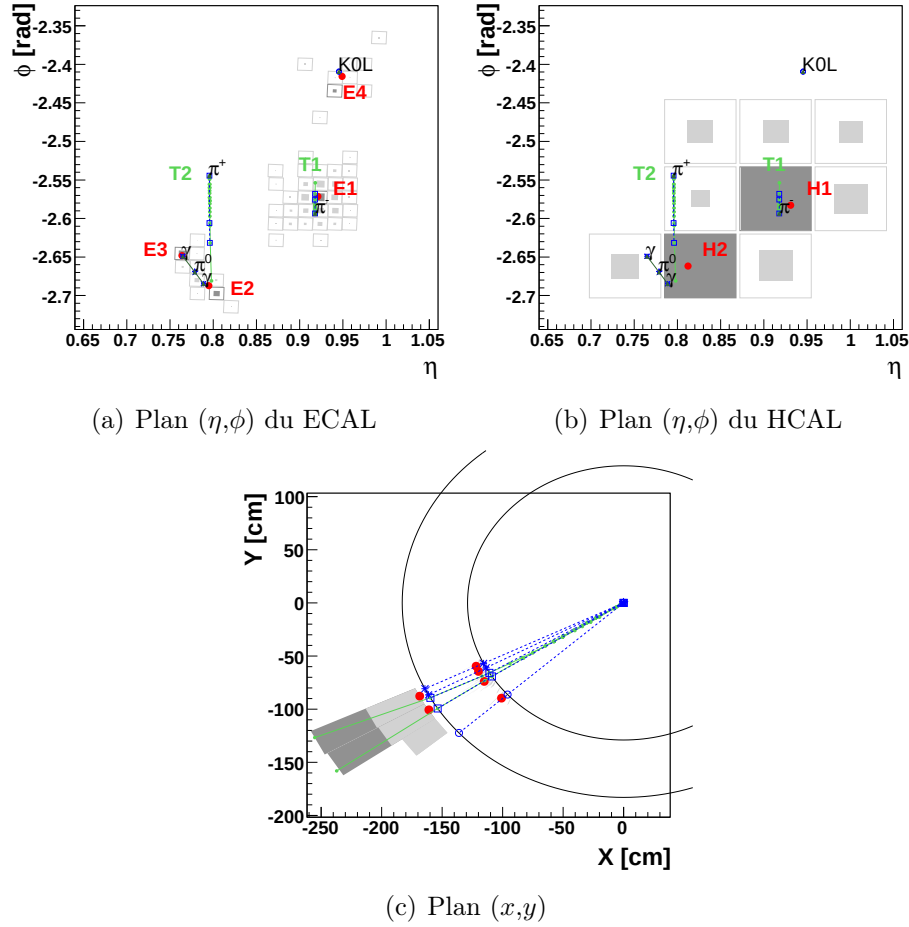
FIG. 4.19 – Vue sch matique d'un jet hadronique dans le plan (\eta, \phi) et dans le plan (x, y) . Le jet est compos  d'un K_L^0 , d'un \pi^- , d'un \pi^+ et d'un \pi^0 se d sint grant en deux photons.
