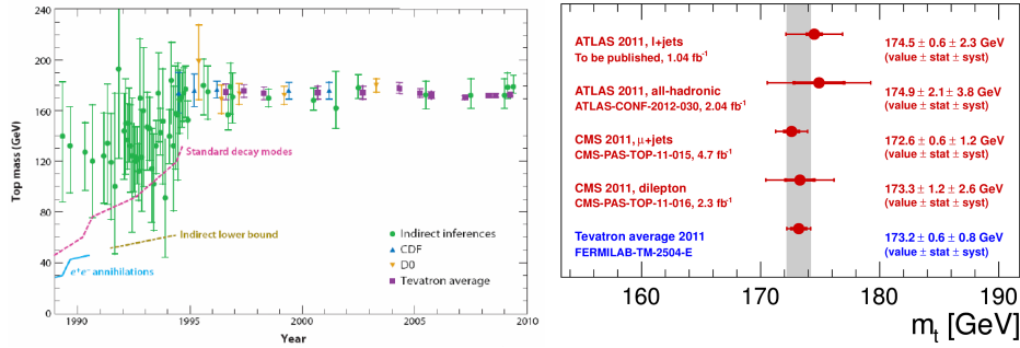
FIG. 2.1 – A gauche est représentée l'évolution de la masse du quark top en fonction du temps [23]. A droite sont représentées les dernières mesures officielles des expériences CMS, ATLAS et Tevatron sur la masse du quark top [24].
