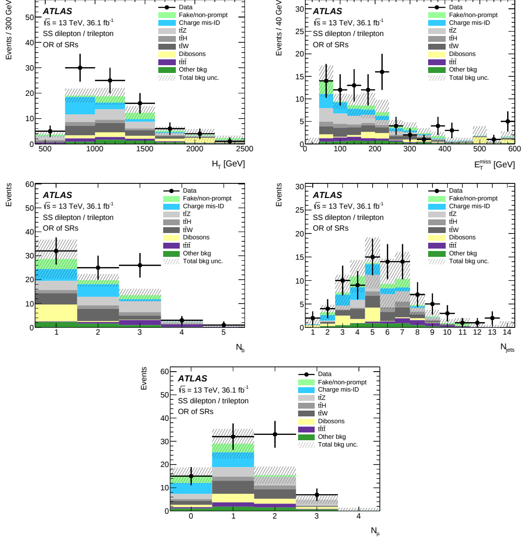
Figure 5.13 – Distributions de variables cinématiques des événements entrant dans n'importe quelle région de signal. De gauche à droite puis de haut en bas les variables sont H_T , E_T^{\text{miss}} , le nombre de jets de quarks b N_b , le nombre de jets N_{\text{jets}} , et enfin le nombre de muons N_{\mu} .
