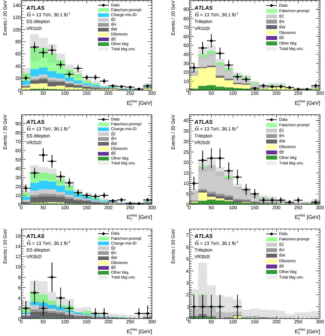
Figure 5.5 – Distributions de la grandeur E_T^{\text{miss}} dans les régions de validation. De haut en bas il s'agit des régions 1b, 2b, puis 3b. Les régions 2 \ell sont à gauche, et les régions 3 \ell à droite. Les histogrammes colorés empilés représentent l'estimation des bruits de fond, et les points noirs sont les données. Les bandes hachurées représentent les incertitudes statistiques et systématiques de l'ensemble des bruits de fond.
