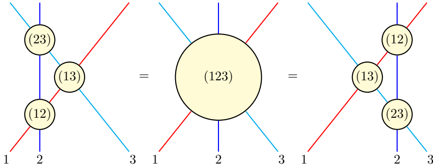
Figuur 1: Een verstrooiingsproces met drie inkomende deeltjes resulteert in drie uitgaande deeltjes (middelste diagram). In een integreerbare theorie kan dit proces worden beschreven als twee verschillende opeenvolgingen van verstrooiingen van twee deeltjes, die equivalent horen te zijn. Dit is een niet-triviale conditie op de S-matrix van twee deeltjes.
