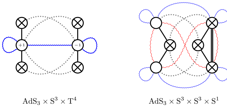
Figuur 2: Een grafische weergave van de kwantisatiecondities op de impulsen van deeltjes (Bethe-Yang vergelijkingen). De verschillende soorten deeltjes worden weergegeven door de knopen in het Dynkin diagram van de supersymmetrie algebra van beide theorieën ( \mathfrak{psu}(1, 1|2)^2 en \mathfrak{d}(2, 1; \alpha)^2 respectievelijk). De lijnen geven verscheidene interactietermen in de Bethe-Yang vergelijkingen weer.
